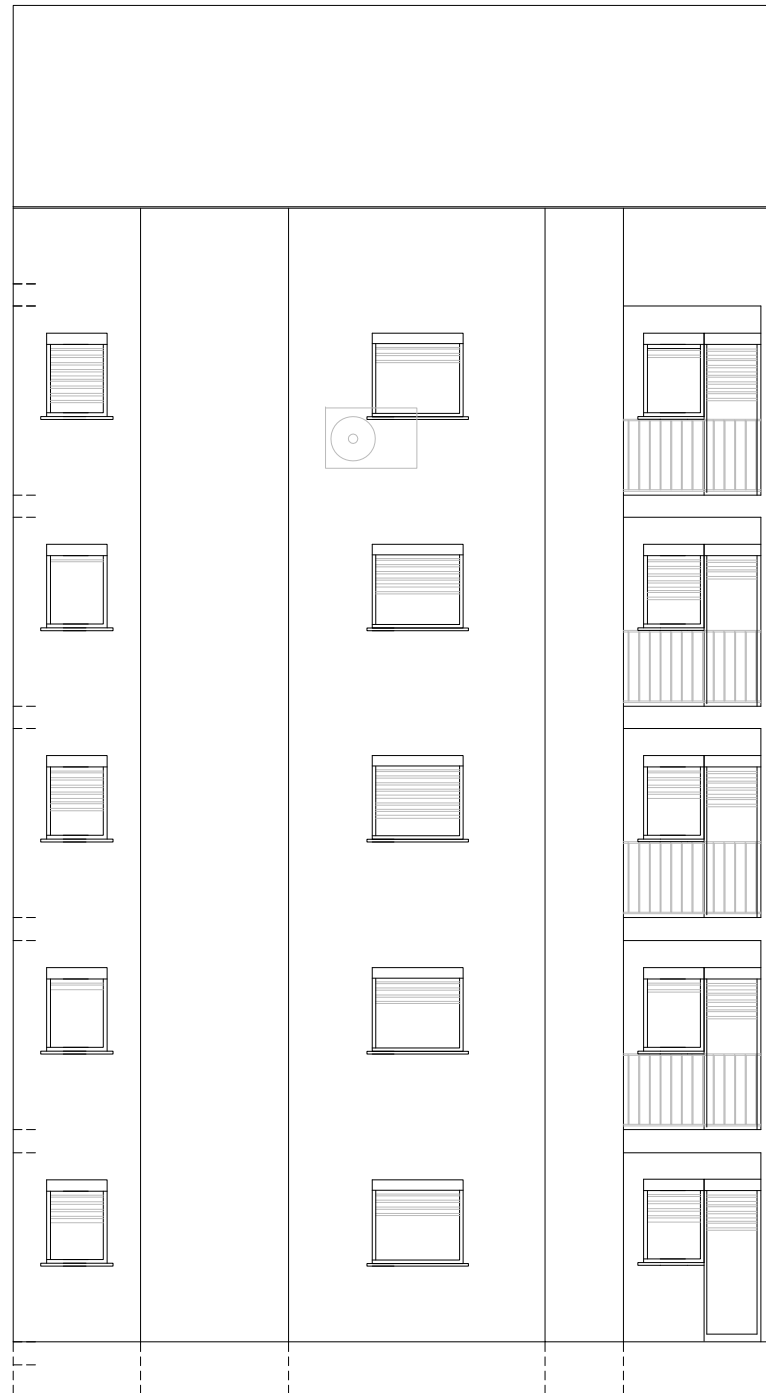
DESENVOLUPAMENT FAÇANA POSTERIOR
