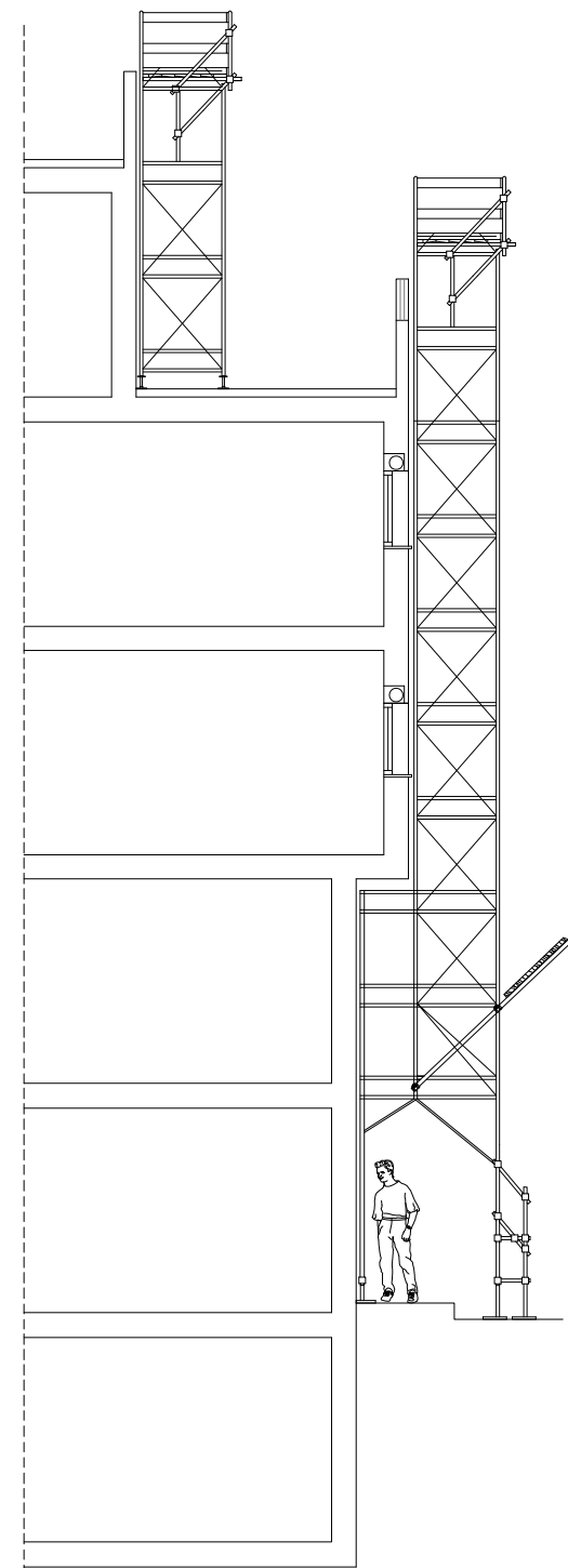
SECCIÓ FAÇANA PRINCIPAL
