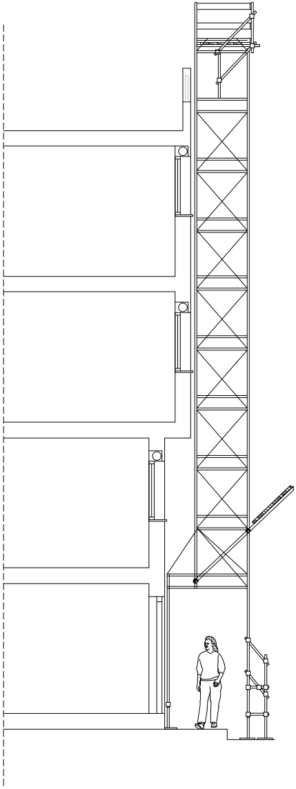
SECCIÓ FAÇANA PRINCIPAL
