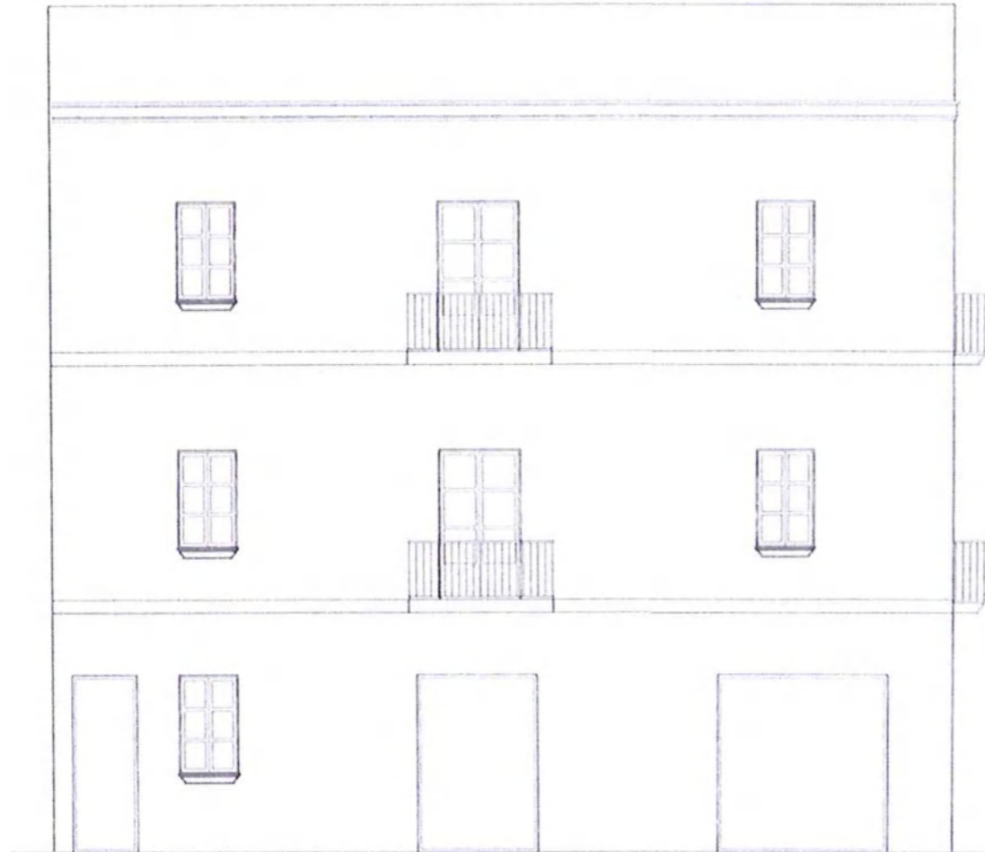
Façana c. Vistalegre (any 1.999)
