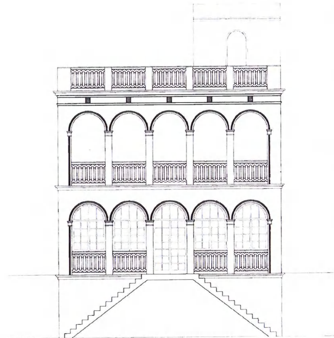
Façana jardí posterior
