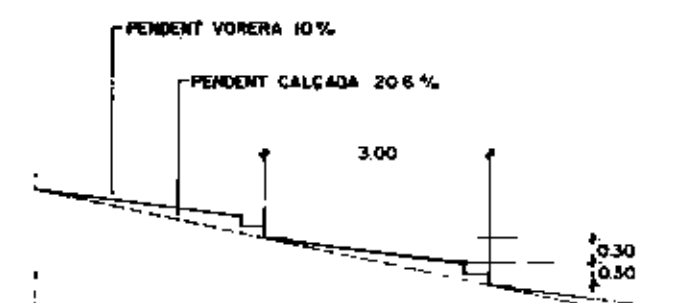
DETALL SECCIO DEL NOU CARRER E 1/100
